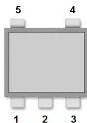
Fig3 SOT553
